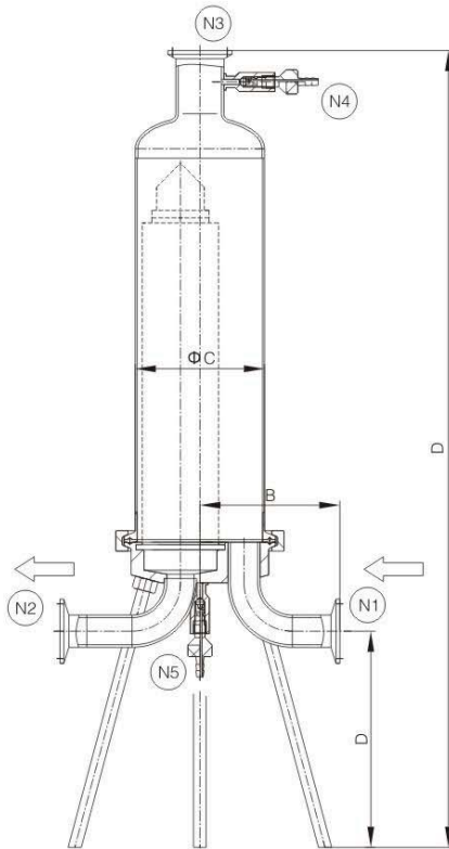
单芯卫生级液体过滤器(222型、226型) Single fluid sanitary filter housing(222type、226type)
